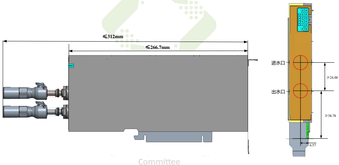
图3 结构设计要求（流体快插接头位于加速卡尾部）
